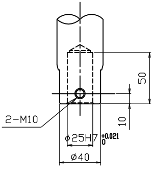
ラム寸法図
